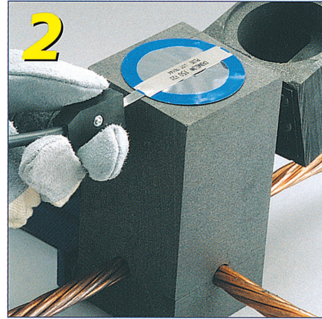
Adım 2: Ateşleme şeridine elektronik ateşleyici bağlanır.
